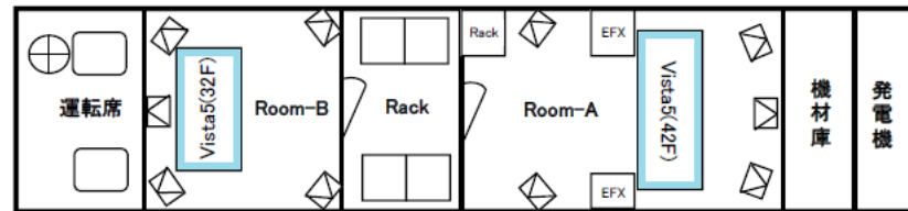
内観図
